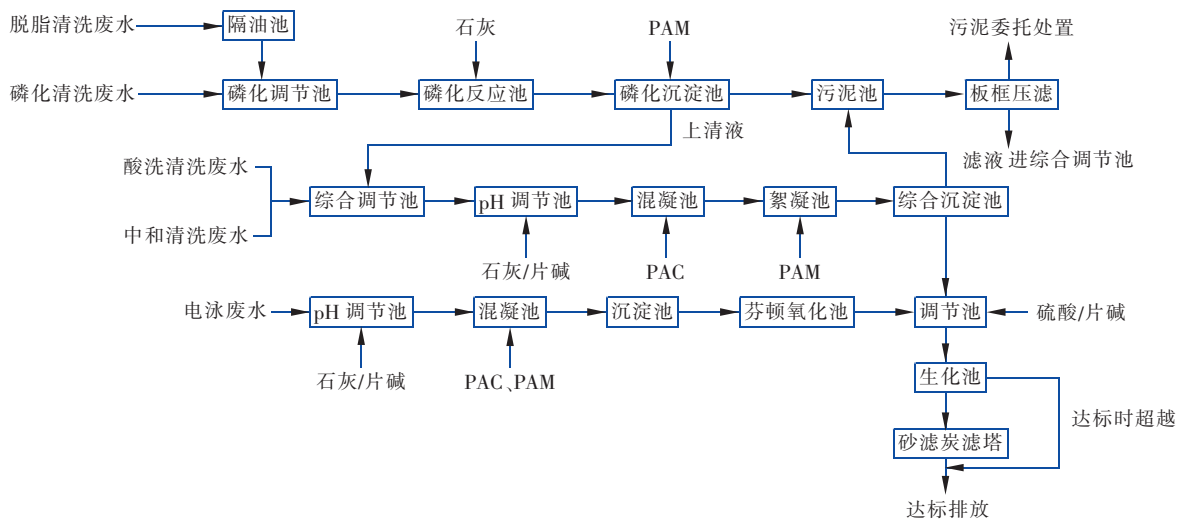
图 1 改造后的废水处理工艺流程
