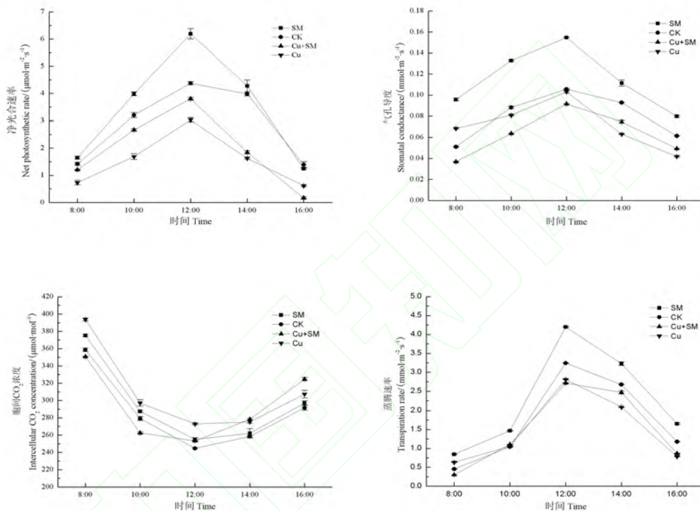
图 2 接种土壤微生物对 Cu 胁迫下海州香薷叶片净光合速率( P_n )、气孔导度( G_s )、胞间 \text{CO}_2 浓度( C_i )、蒸腾速率( T_r )日变化的影响
