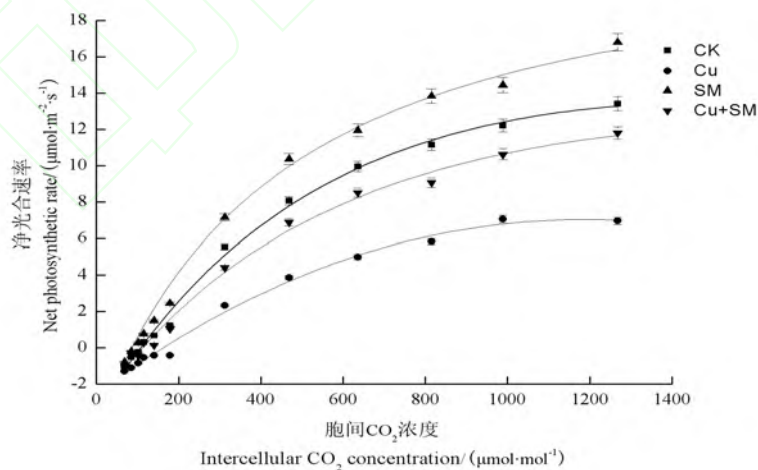
图 4 接种土壤微生物对 Cu 胁迫下海州香薷光合- \text{CO}_2 响应曲线的影响
