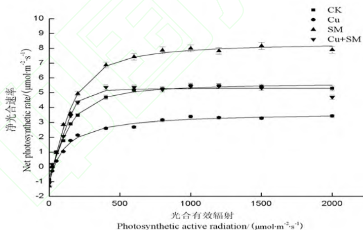
图 3 接种土壤微生物对 Cu 胁迫下海州香薷光合-光响应曲线的影响
