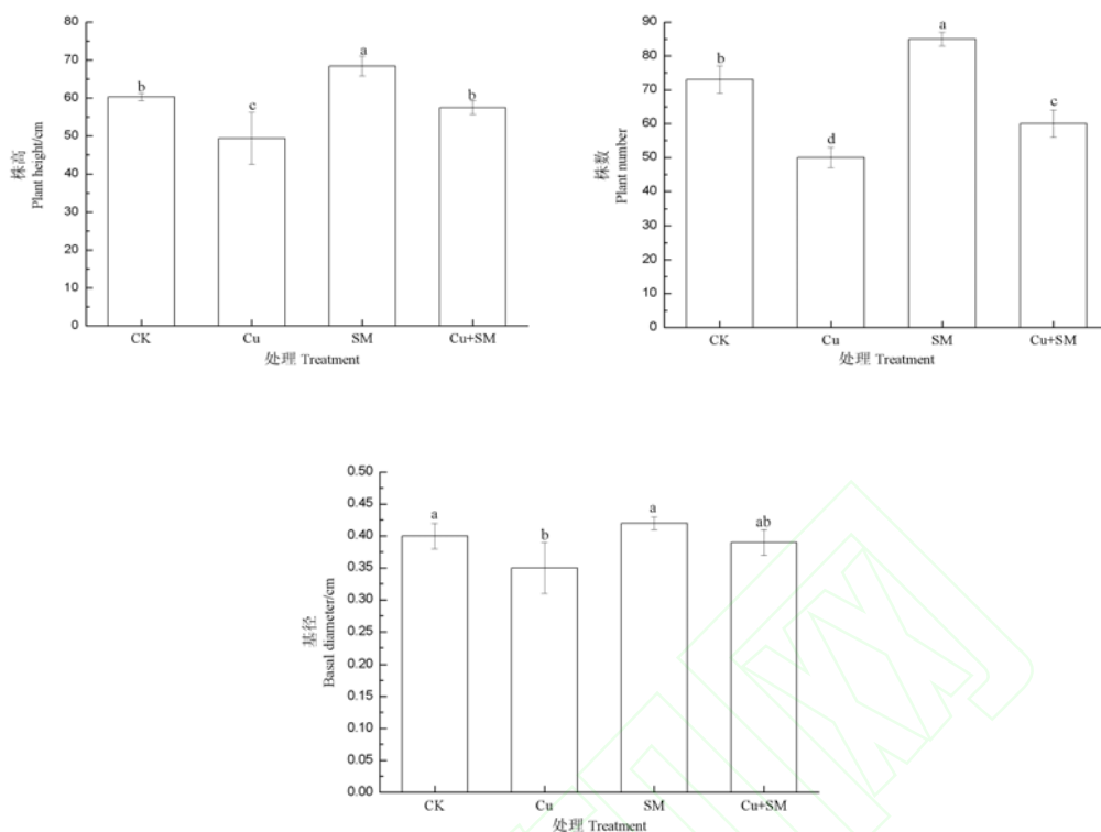
图 1 接种土壤微生物对 Cu 胁迫下海州香薷生长的影响
